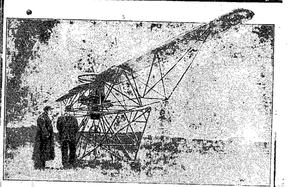
Hierboven een uitvinding van den Duitschen ingenieur Zeschka. Het is een vliegtuig dat door middel van een groote schroef met gewelddige vleugels loodrecht naar boven kan stijgen en evenzoo dalen.
